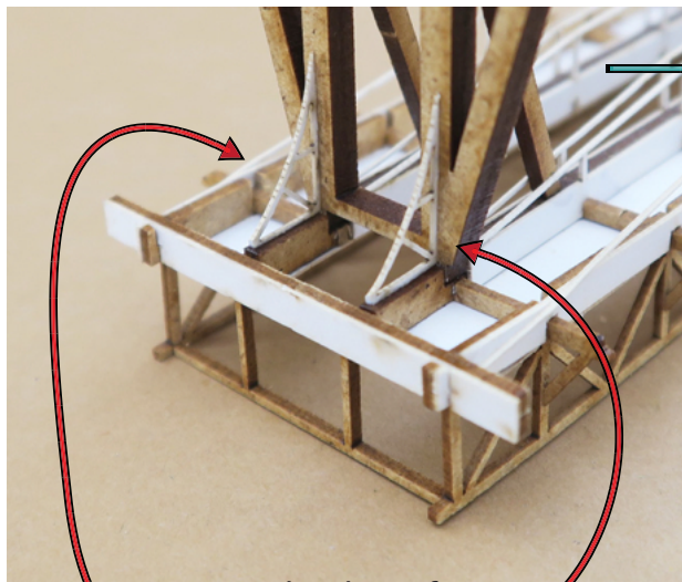
Consoles de renfort
